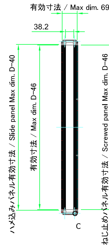
B-B ( 1 : 10 )
